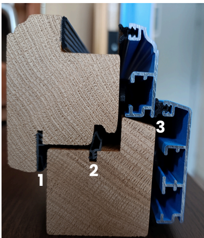
Trois joints d'étanchéité
