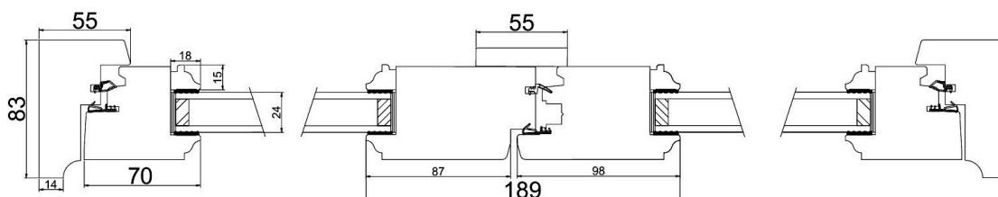
Coupe horizontale pour porte-fenêtre 2 vantaux avec serrure et verrou haut et bas sur semi fixe
