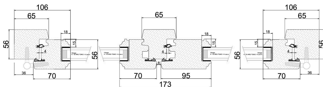
Coupe horizontale pour porte-fenêtre 2 vantaux avec serrure et crémone sur semi fixe
