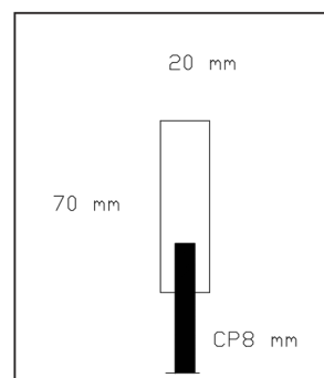
Cadre 20mm et contreplaqué ébénisterie (8mm)
