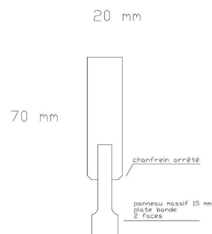
Cadre 20mm et panneau massif platebande (15mm)
